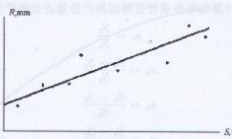
图 E.2 R - S 关系图
