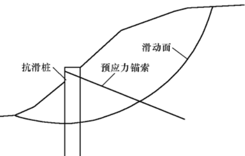
图2 钢筋混凝土抗滑桩式锚杆挡墙
