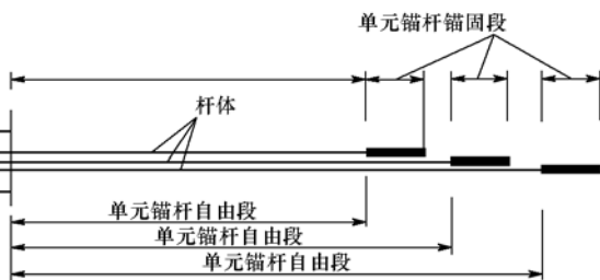
图8 拉力分散型预应力锚杆结构原理图
