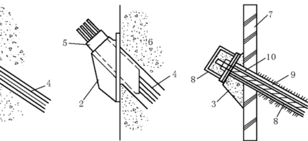
图 10 锚头及传力结构示意图
