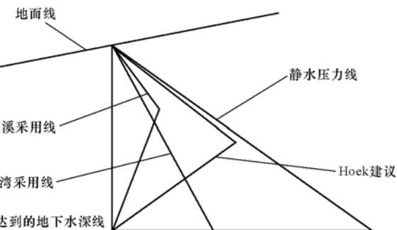
1 各工程采用的因降雨而形成孔隙压力分布图
