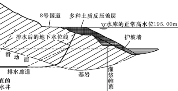
新西兰 Clyd 水电工程 Brewery Creek 滑坡加固工程
