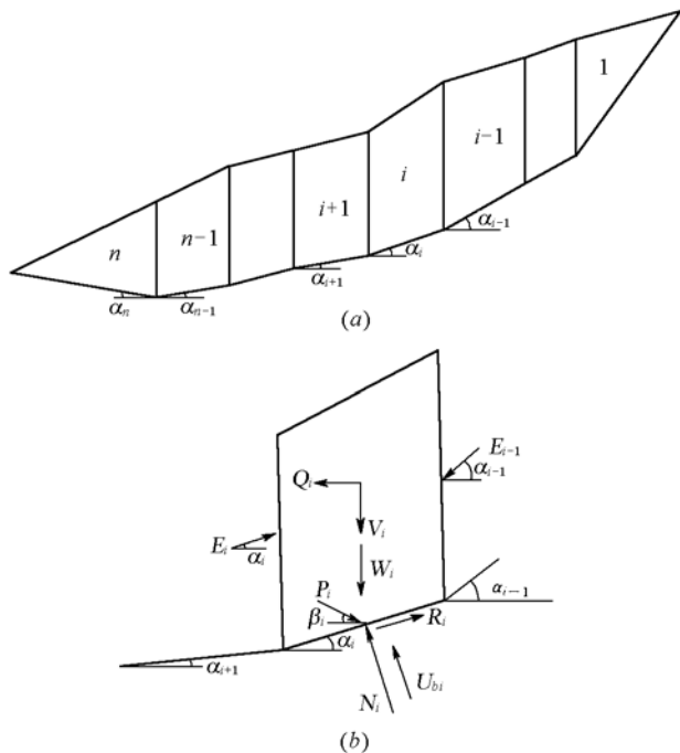
图 D.1.3 不平衡推力传递法计算简图
