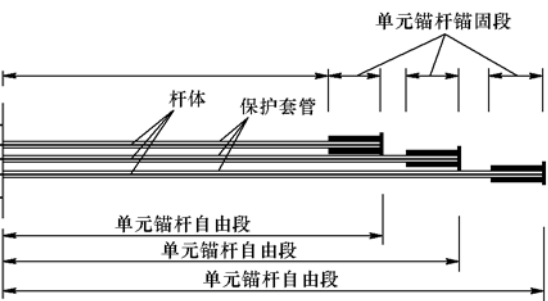
图9 压力分散型预应力锚杆结构原理图
