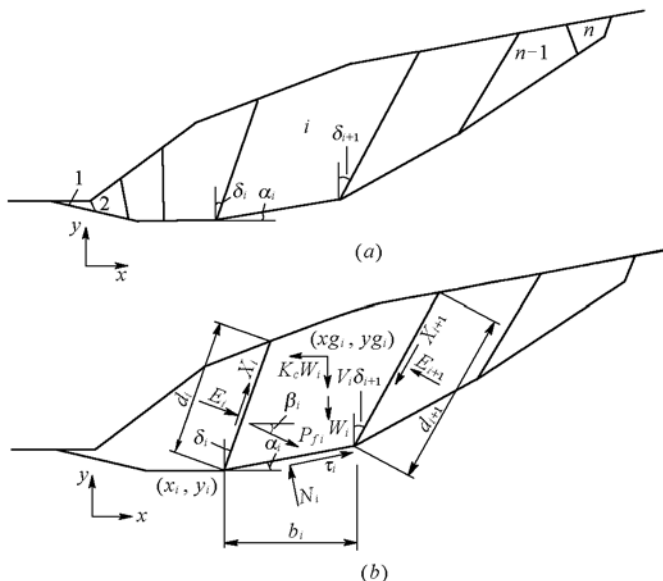
图 D.1.4-1 Sarma 法计算简图
