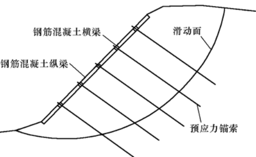
图3 钢筋混凝土格构式锚杆挡墙
